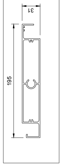
195 LOUVER BLADE DETAIL SCALE 1:2 @A1
